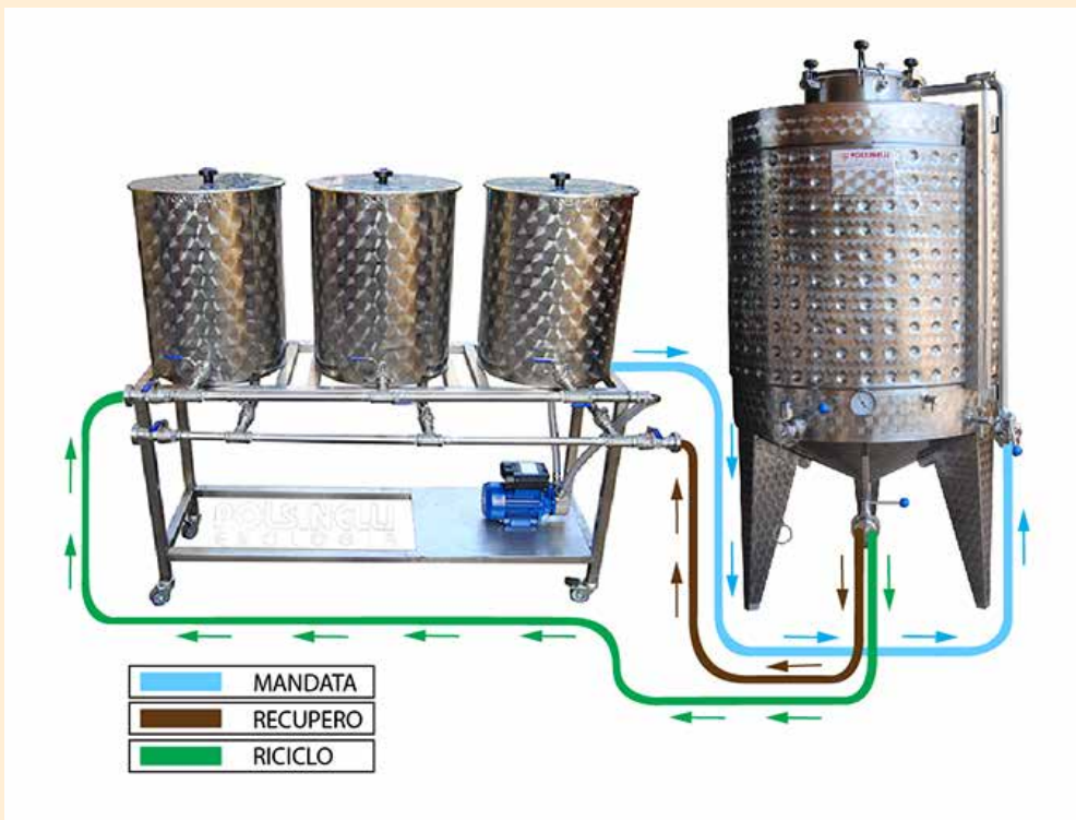
SISTEMA DI LAVAGGIO AUTOMATICO A PRESSIONE
